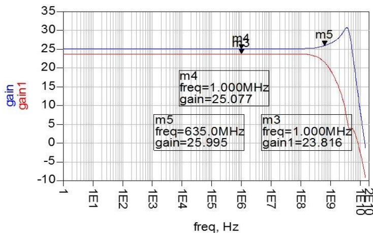
شکل ۷: نتیجه شبیه سازی بهره طبقات تقویت کننده
